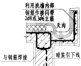
挑檐内暗装
