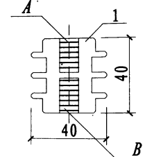
1-1剖面图
