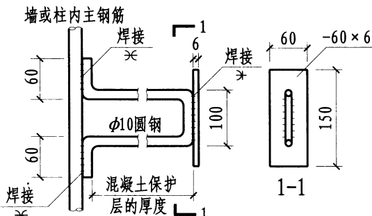
预埋连接板做法1
