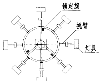
灯盘俯视图
