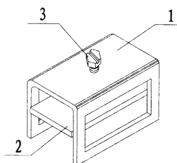
TE-2透视图
