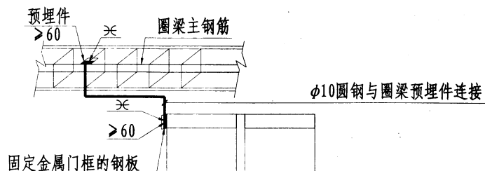
金属门框防侧击雷做法
