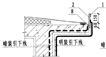
挑檐上明装 I
