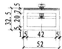
TE-1 ~ TE-4正视图
