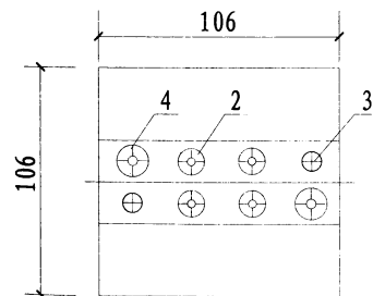
俯视图
