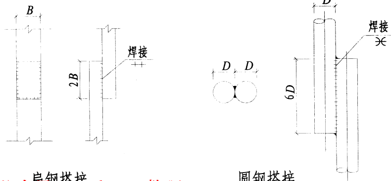
扁钢搭接
