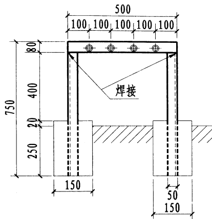
接地端子板
