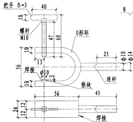
移动接地线夹
