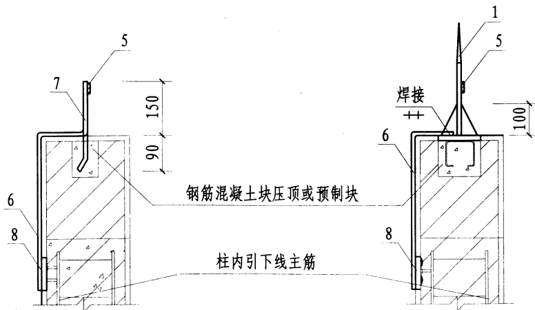
2-2剖面图
