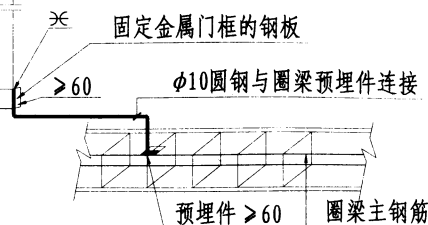
金属门框防侧击雷做法
