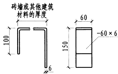
① 引出连接板大样
