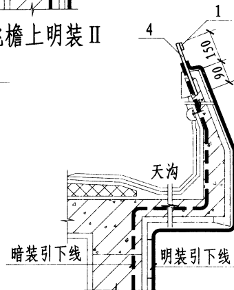
挑檐上明装 V
