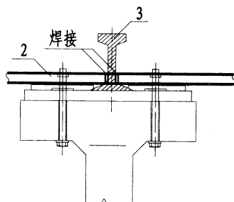
I型重轨
