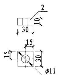
垫片
