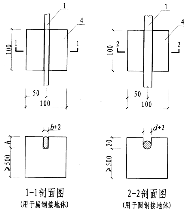
III 型支持器
