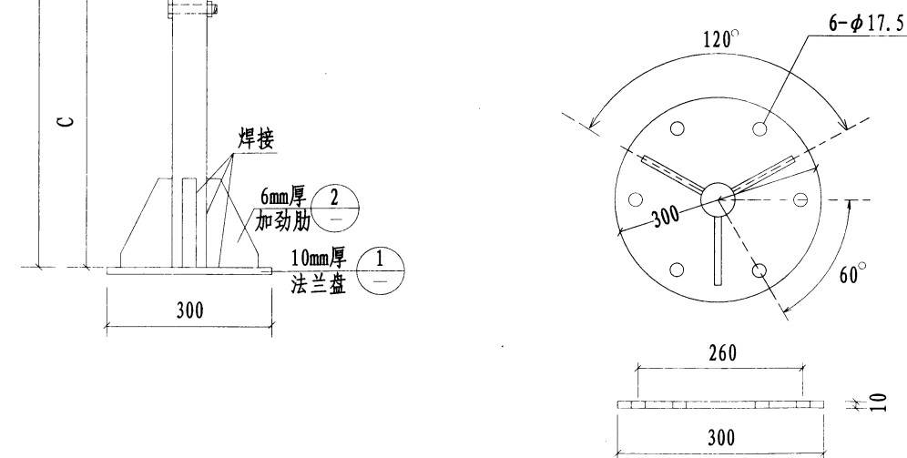
1 法兰盘
