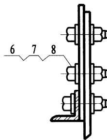
2-2剖面
