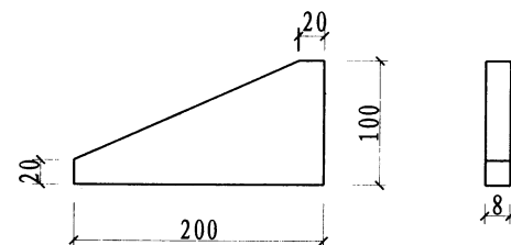
2号零件
