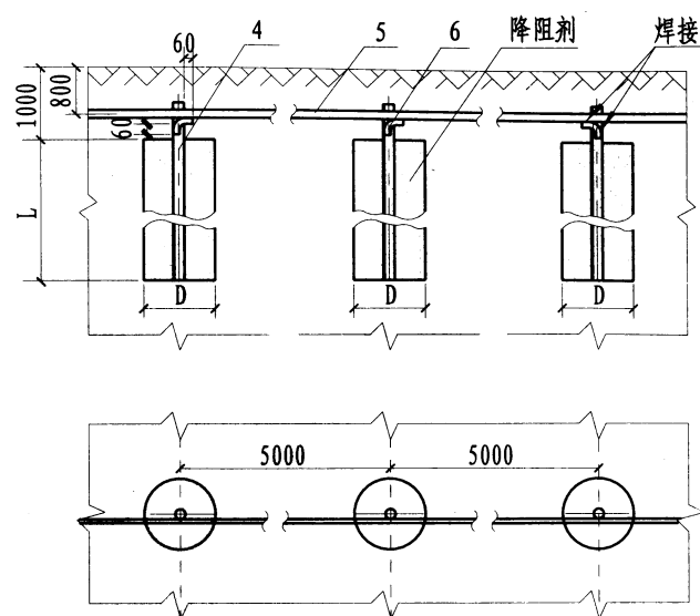
圆钢接地体
