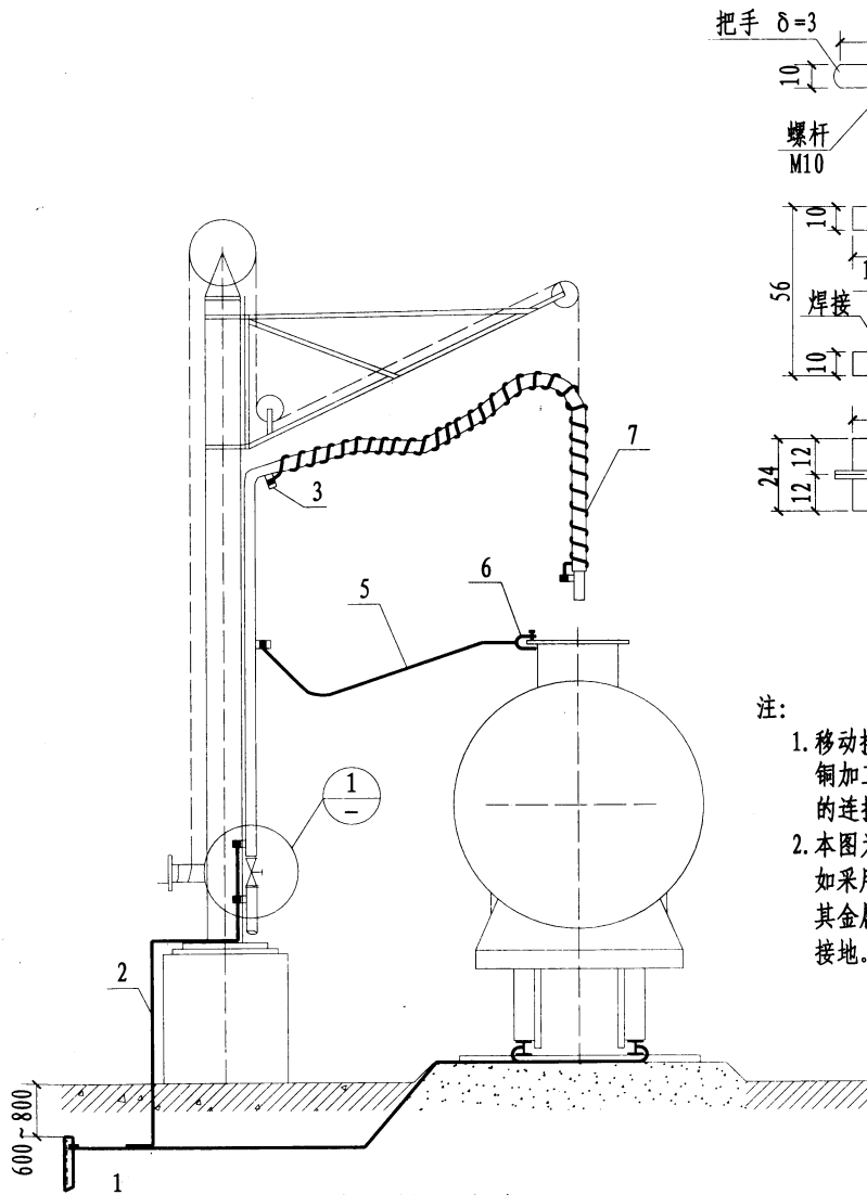
移动接地线夹
