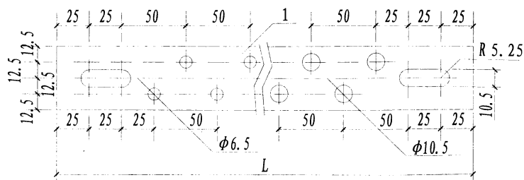
端子板长度表
