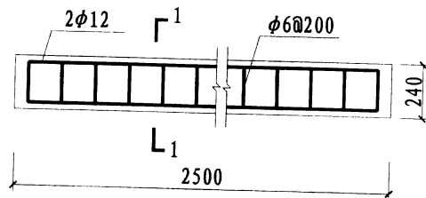
梁钢筋图
