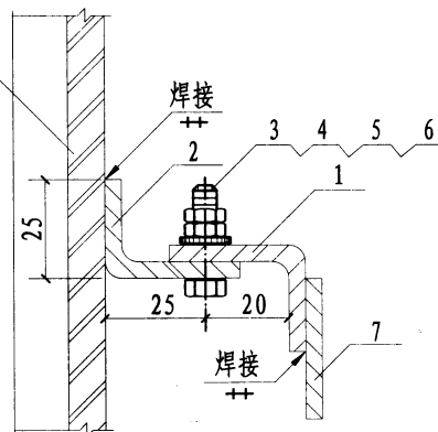
金属外壳接地
