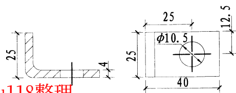
连接耳
