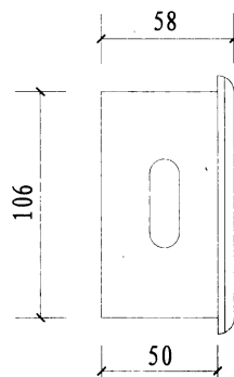
侧视图
