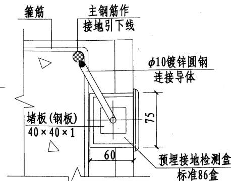
1-1剖面图
