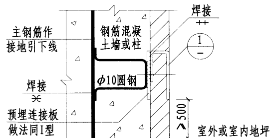
预埋接地连接(检测)板
