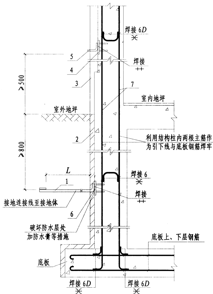
① 有防水层防雷引下线外引做法
