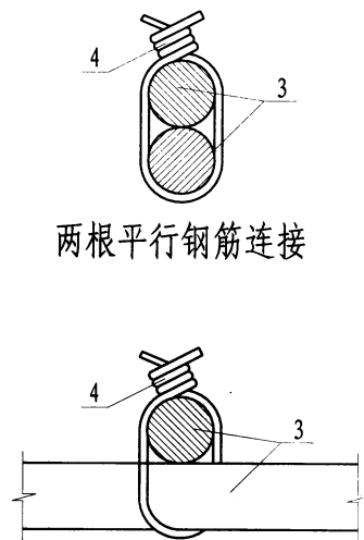
(二) 绑扎连接
