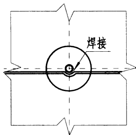
钢管接地体
