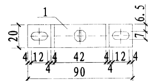
俯视图
