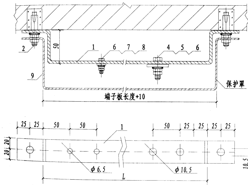
端子板与连接线的连接
