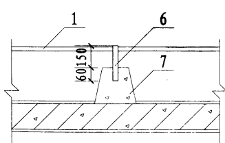
屋面上明装 II
