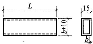
方套管
