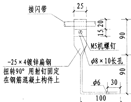
② 斜脊瓦支持卡做法
