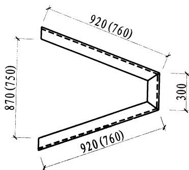
2号零件
