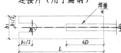
连接片 (用于圆钢)
