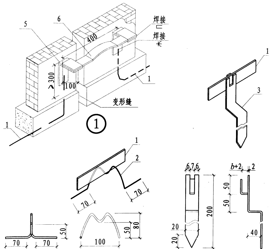
II 型支持器
