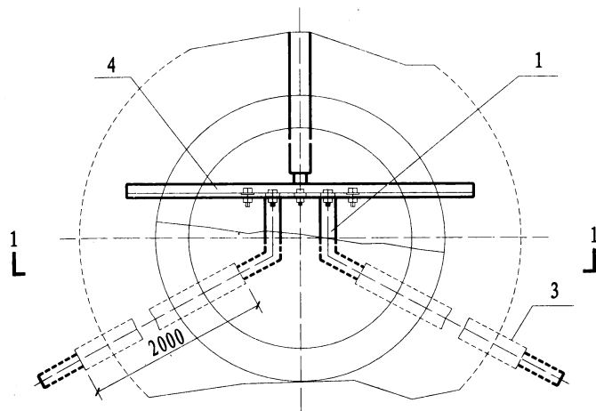
检测井平面图
