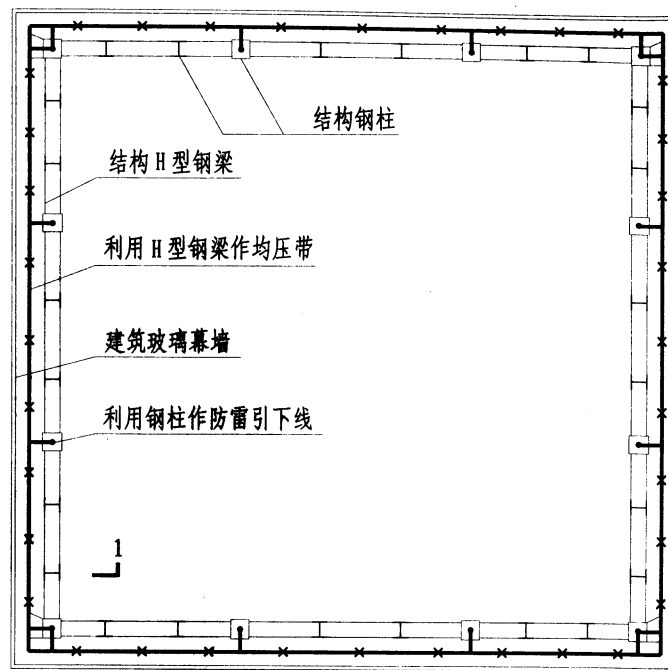
楼层平面图
