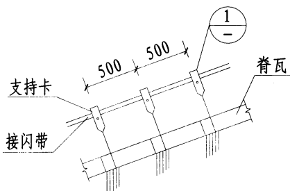
斜脊接闪带做法
