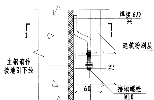
① 钢筋混凝土柱(墙)上安装做法
