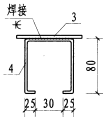
3、4号零件
