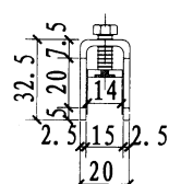
TE-3侧视图
