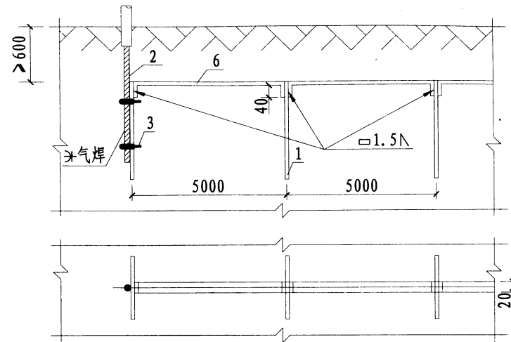
接地体安装
