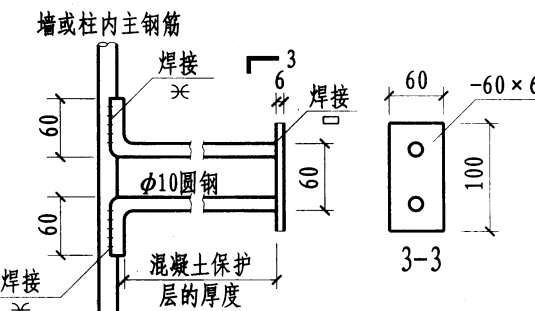
预埋连接板扁钢做法
