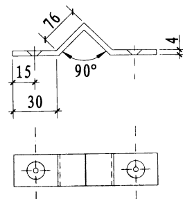
卡子
