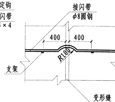
接闪带过变形缝做法 III
